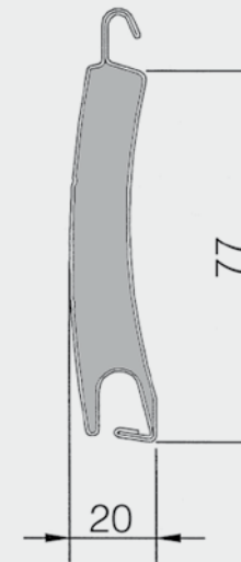
Profil d'une lame isolée
